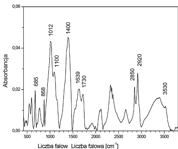
Wykres 2. Wynik analizy próbki (nr 3) warstwy malarskiej wraz z zaprawą metodą spektroskopii w podczerwieni spektrometrem FTIR. Pasma absorpcji potwierdzające obecność: czerni węglowej, oleju lnianego, kredy, kleju glutynowego (?)
