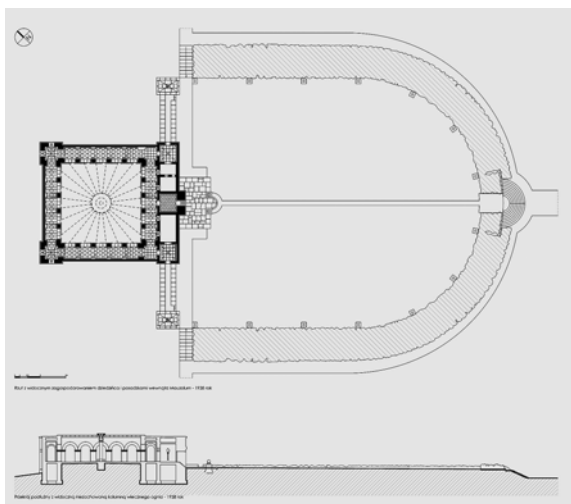
Ryc. 8. Rzut i przekrój pierwotnego założenia Mauzoleum, opracowanie własne na podstawie: „Die Baukunst – Die Kunst im Deutschen Reich”, 1939, nr 1
